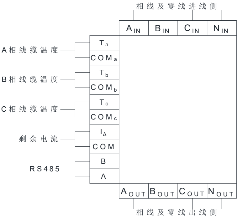
ASCP310 限流式保护器接线端子图
