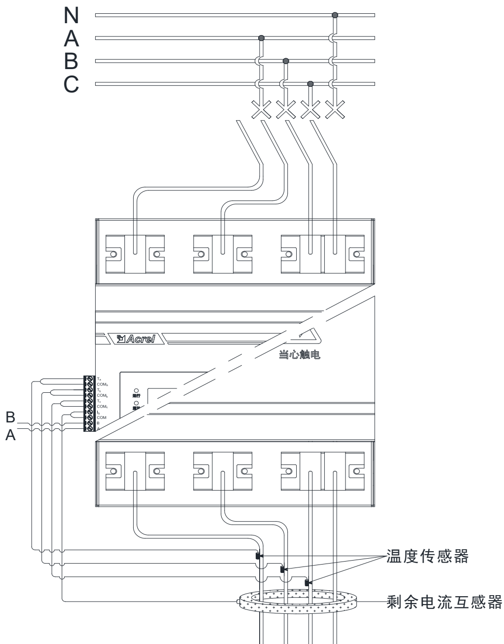
ASCP310 限流式保护器的应用接线图
