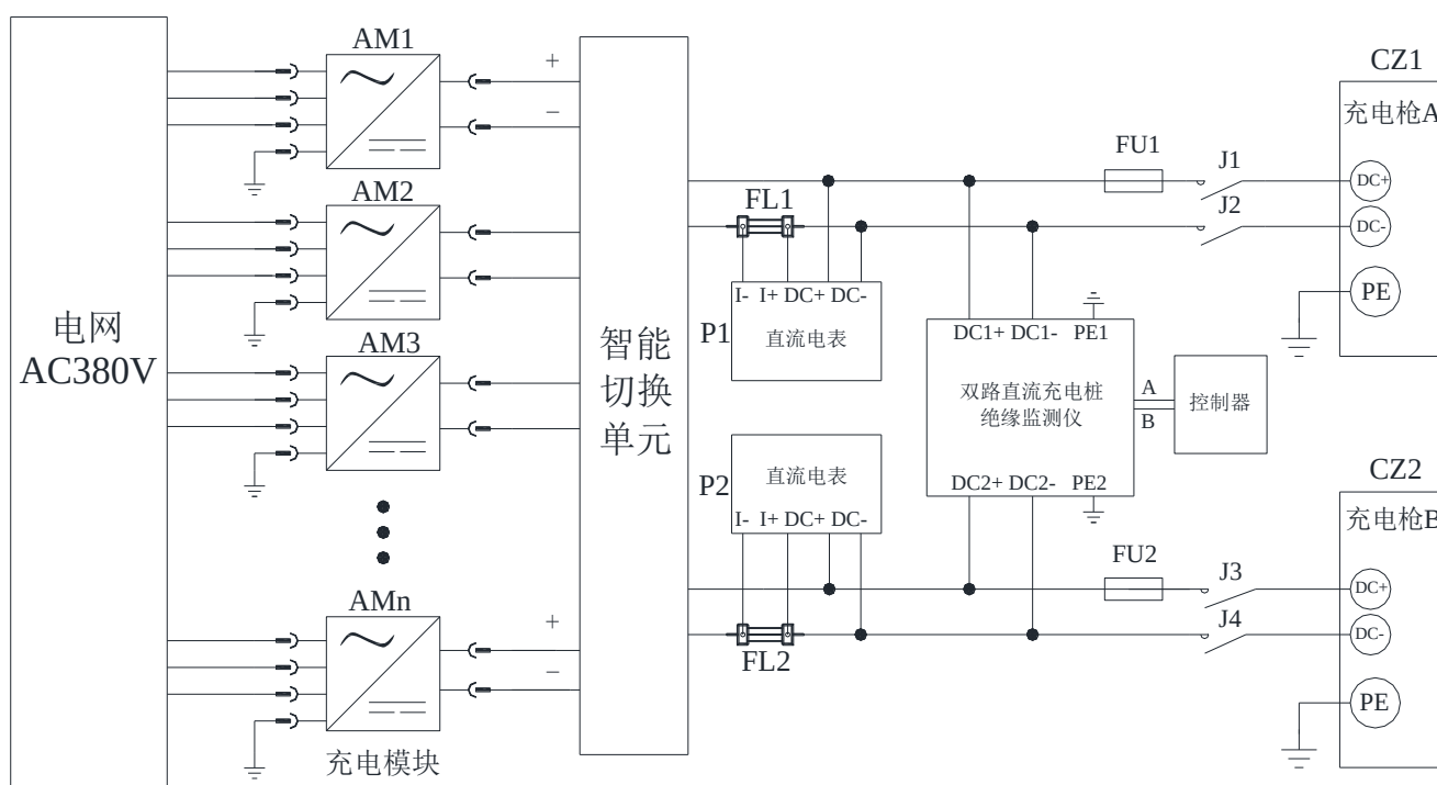
下图为 AIM-D100-CAD 型双路直流充电桩绝缘监测仪在电动汽车直流充电装置中的应用示例。
