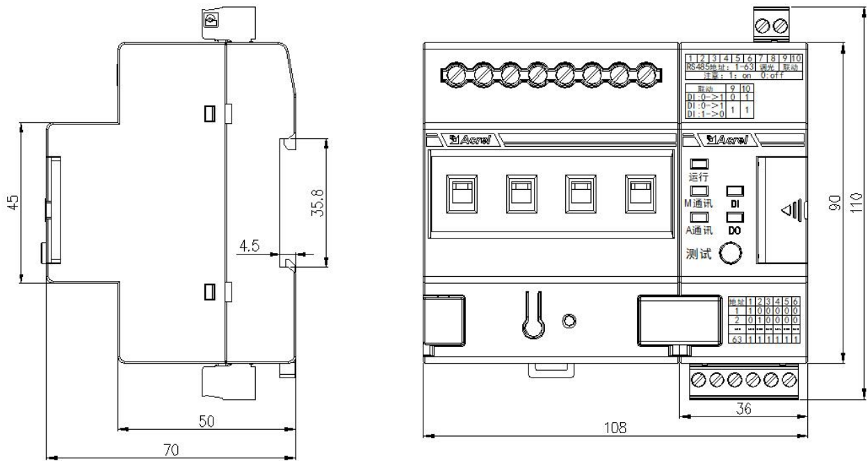
图 2 ASL210-Sx/16 开关驱动器外形及安装尺寸图
