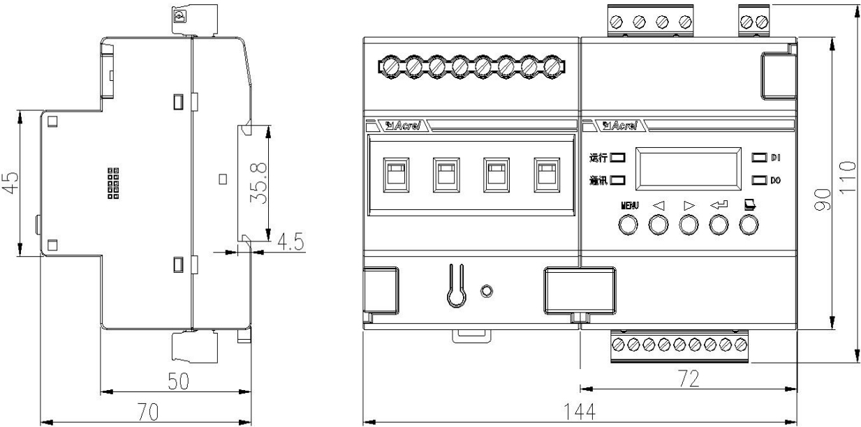
图 1 ASL220Z-Sx/16 开关驱动器外形及安装尺寸图
