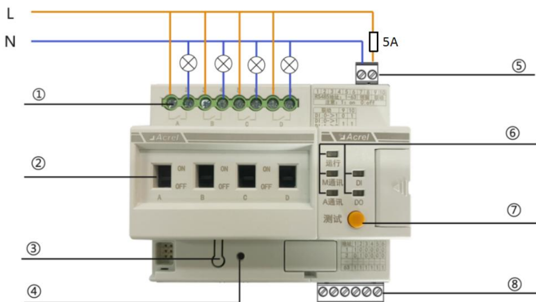
图 4 ASL210-Sx/16 开关驱动器接线示意图
