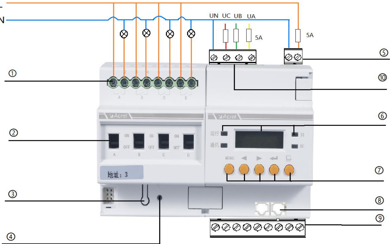
图 3 ASL220Z-Sx/16 开关驱动器接线示意图
