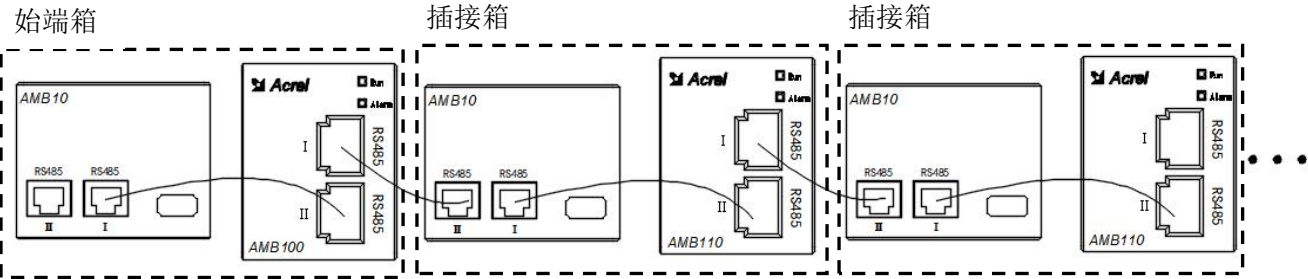
检测模块连接图
