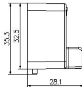
AHKC-BS 霍尔传感器尺寸图
