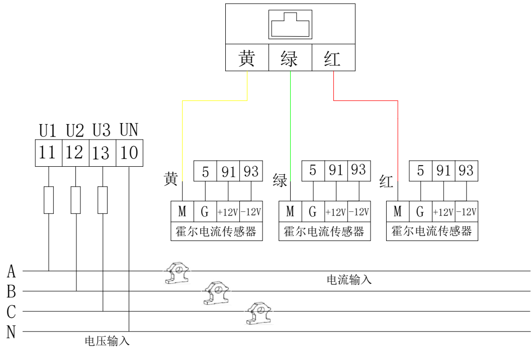
AMB1X0-D(W)-P1 独立辅助电源
