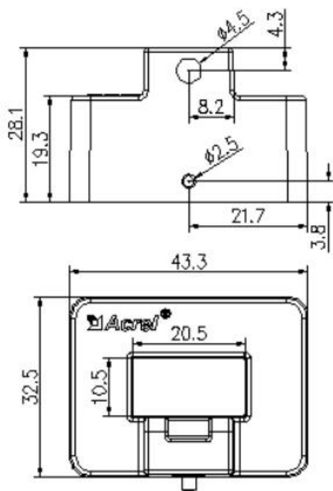
AHKC-BS 霍尔传感器尺寸图
