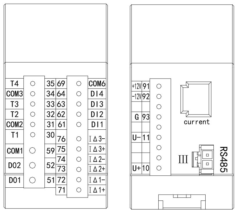
AMB1X0-D(W)信号取电
