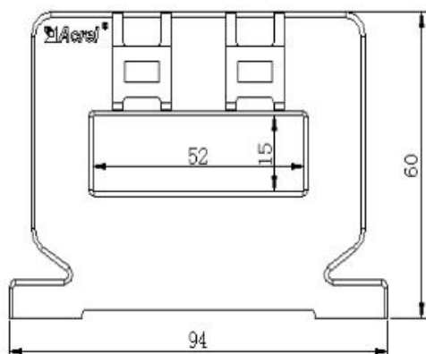
AHKC-FA 霍尔传感器尺寸图
