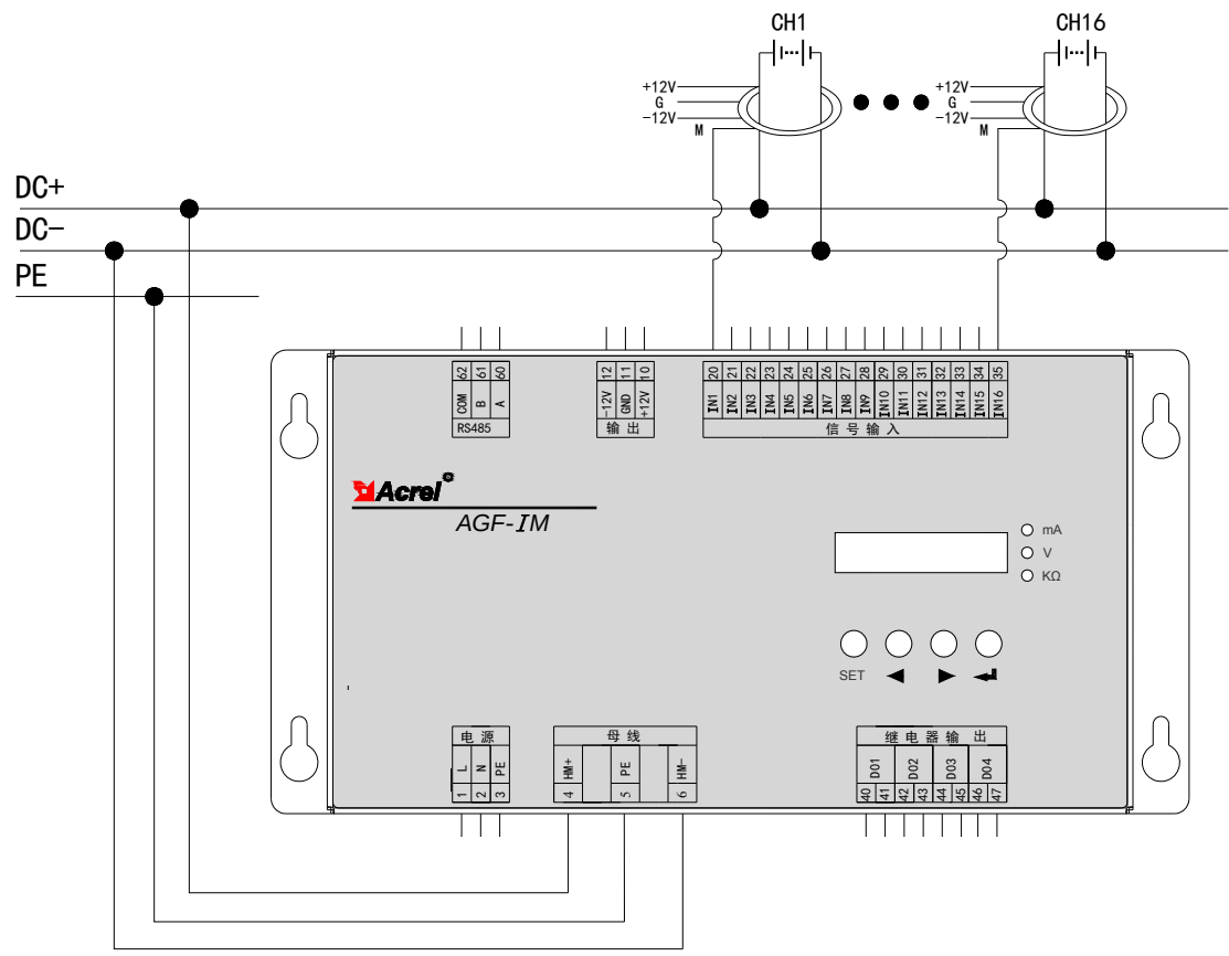
图 2 装置接线图
