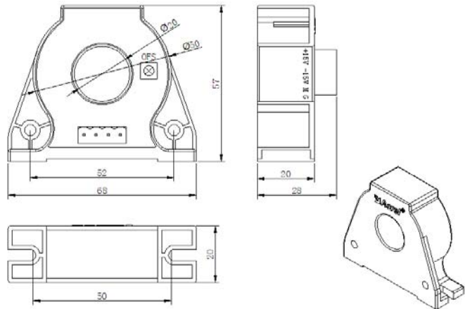
图 4 AHLC-LTA (φ 20) 外形
