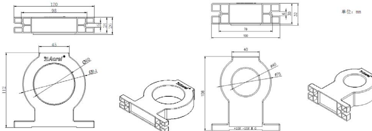
图 2 AHLC-EB (φ 60) 外形
