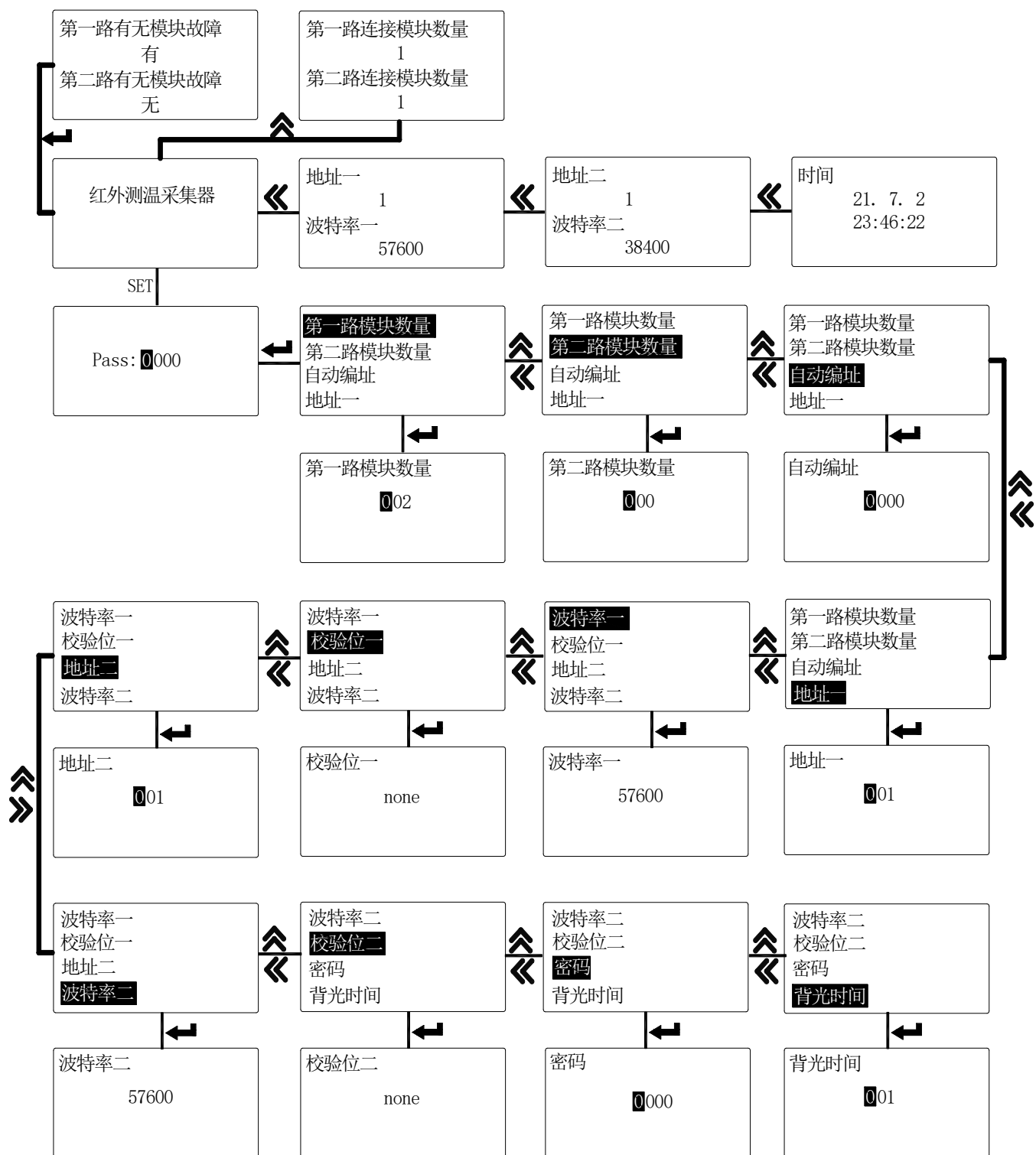
通讯参数选项界面
